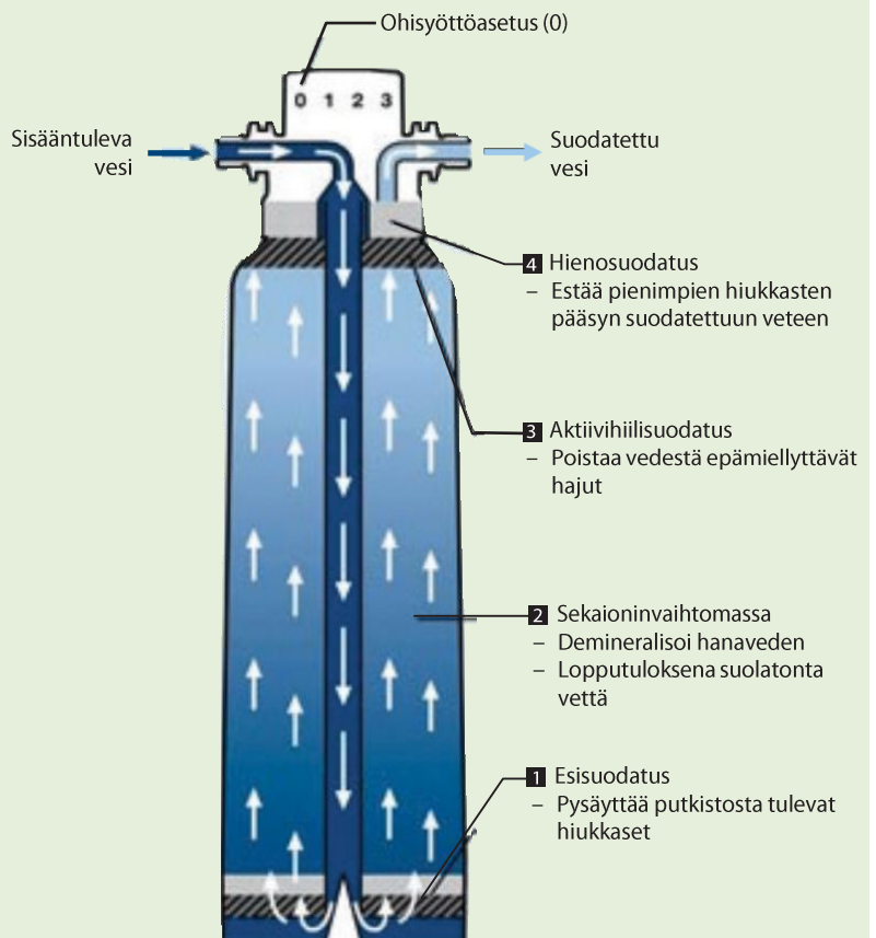
BWT bestdemin PLUS suodattimen rakenne
